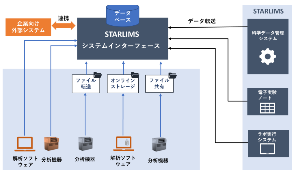
STARLIMS システム構成図
